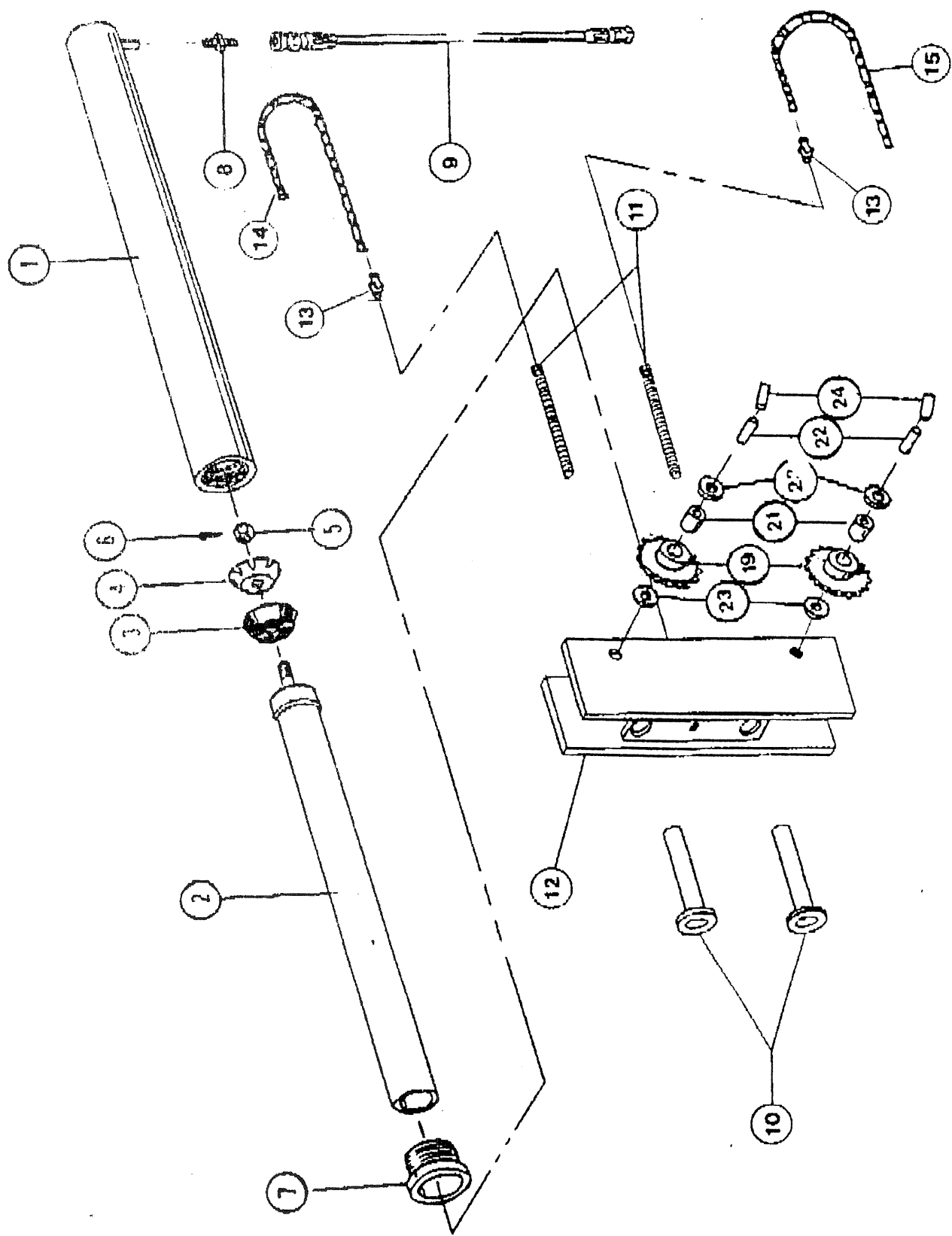
FIG 2a - DD Cylinder Assembly
